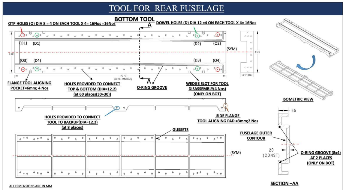
(Item 1.b) Bottom Tool
