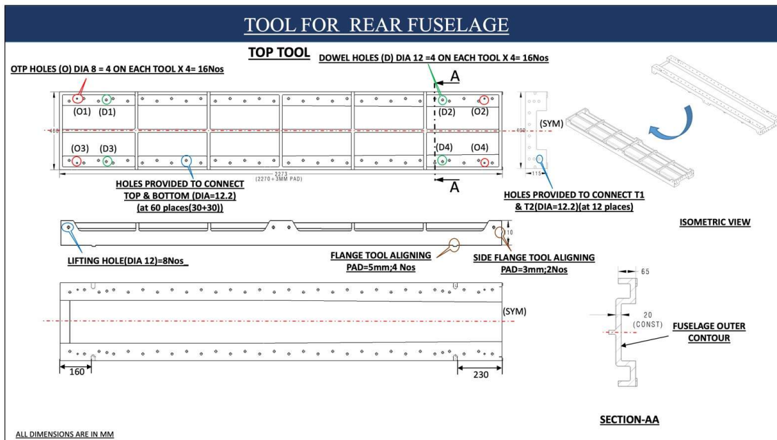
(Item 1.a) Top Tool
