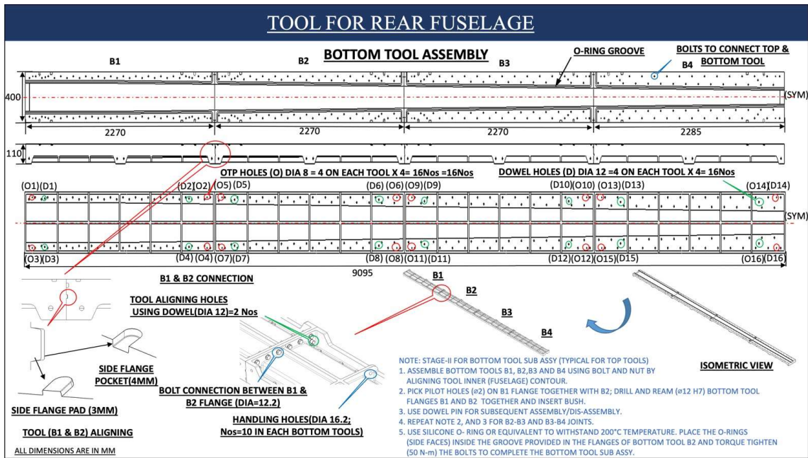
(Item 1.c) Bottom Tool Assembly
