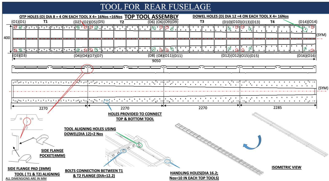
(Item 1.a) Top Tool Assembly
